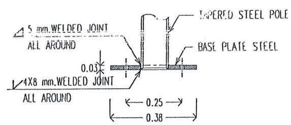
รูปตัด มาตรฐาน
