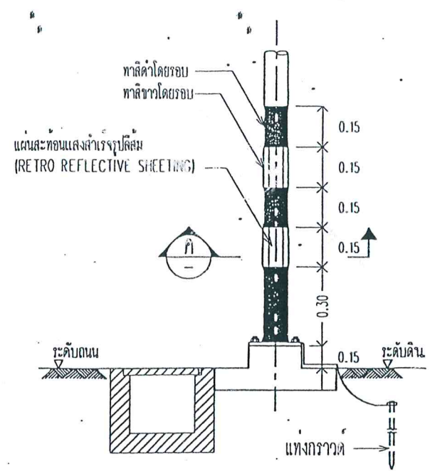
รายละเอียด มาตรฐาน และการติดตั้ง GROUND ROD
